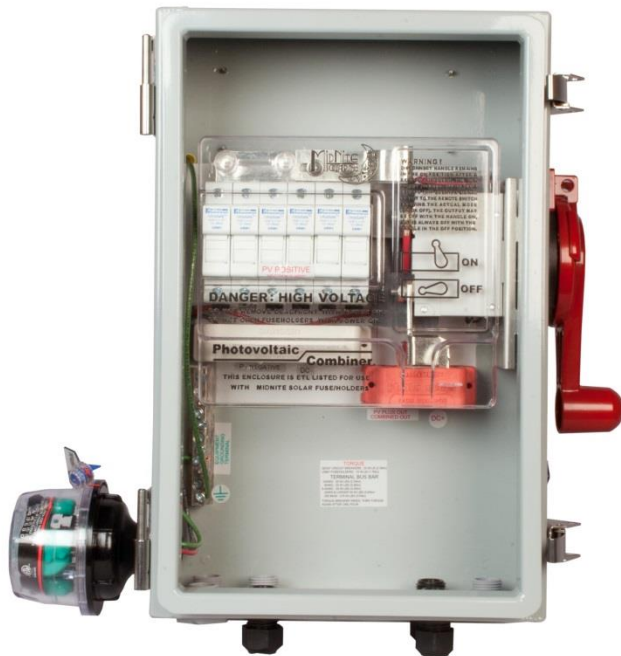
MNPV6HV TYPE 4X
